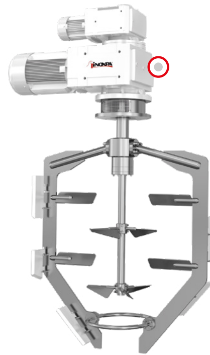
Agitador contrarrotación MCR
